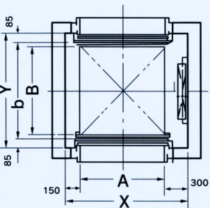
昇降路平面図
