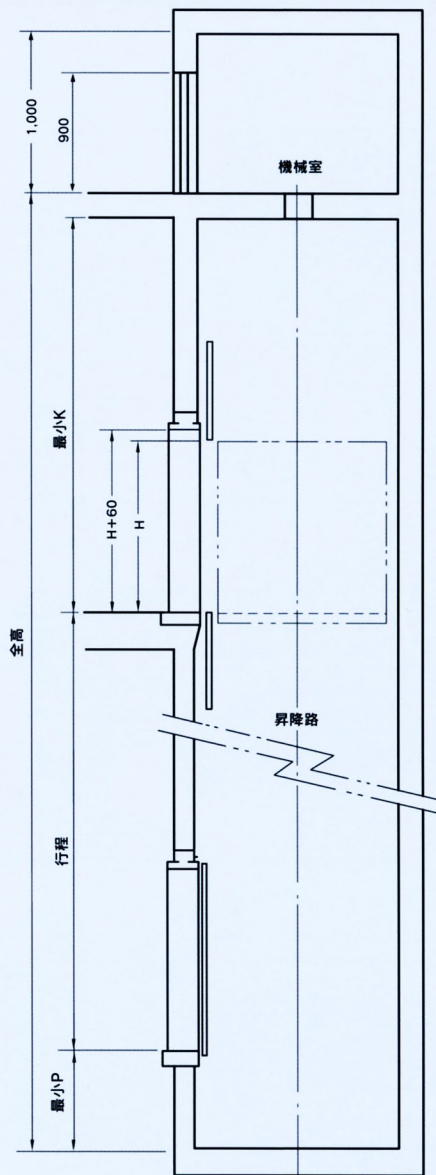
昇降路断面図
