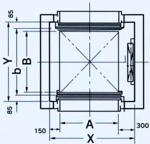
昇降路平面図
